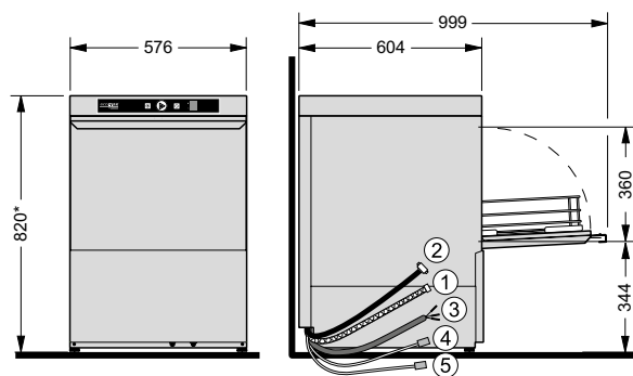
Modell F504 Geschirrspülmaschine
