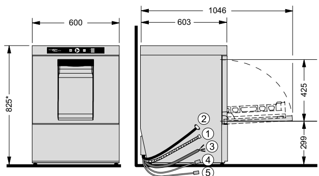
Modell F515 Geschirrspülmaschine
