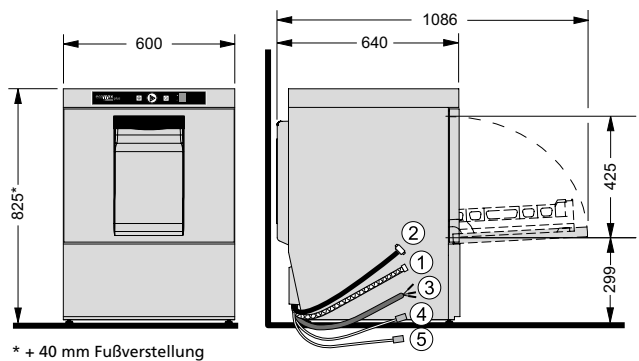
Modell F515L Geschirrspülmaschine
